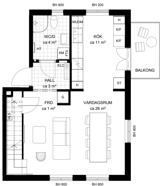
PLAN 1 - ENTRÉPLAN
