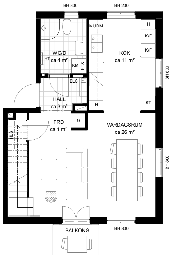
PLAN 1 - ENTRÉPLAN
