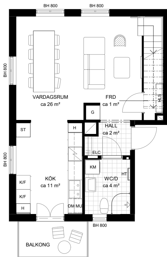
PLAN 1 - ENTRÉPLAN
