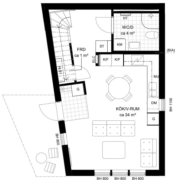
PLAN -1 ENTRÉPLAN
