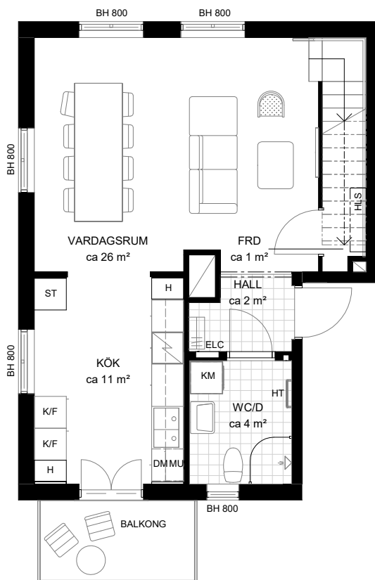
PLAN 1 - ENTRÉPLAN
